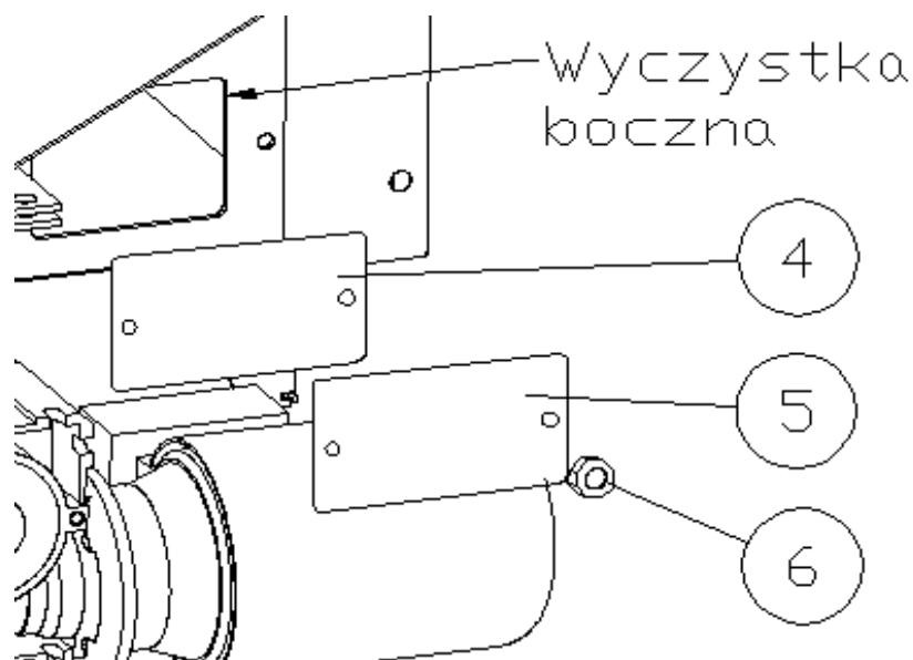
Rys. 10 Czyszczenie kotła przez wyczystkę boczną
