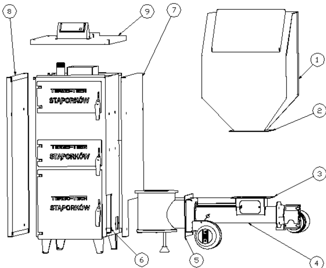
Rys. 12 Przekładanie podajnika na drugą stronę kotła
