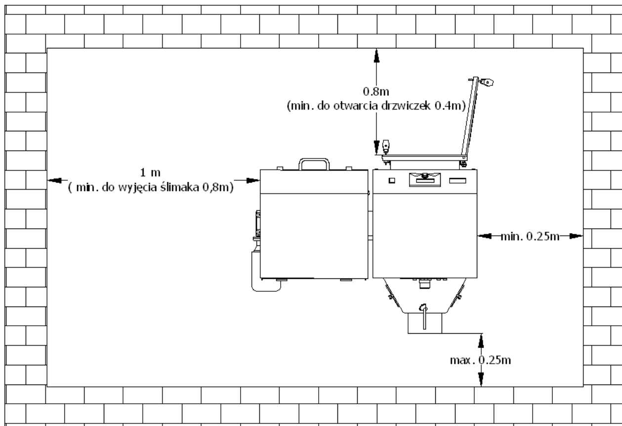
Rys. 2 Usytuowanie kotła w kotłowni
