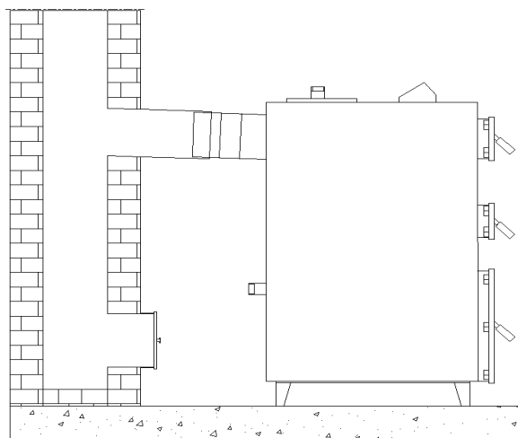
Rys. 3 Podłączenie kotła do komina
