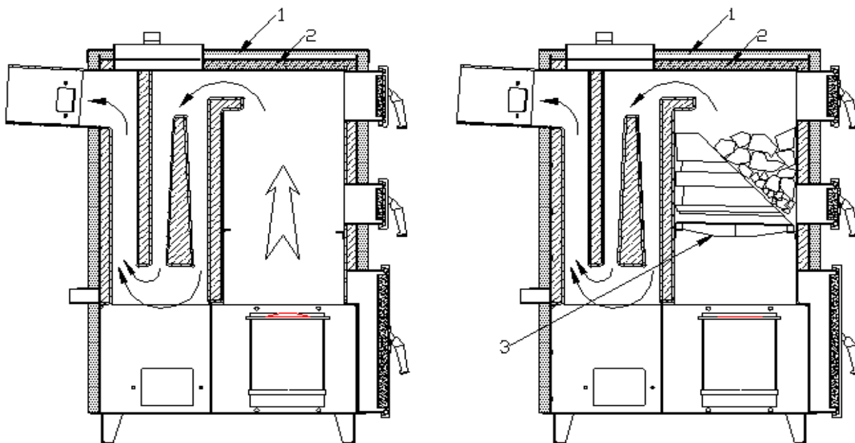
Rys. 8 Przekrój kotła i obiegi spalin przy spalaniu automatycznym (lewy) i ręcznym (prawy)
