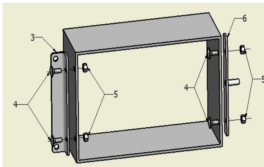
Rys. 14 Mocowanie uchwytów drzwiczek
