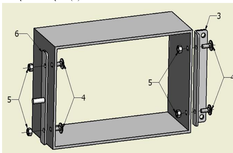
Rys. 15 Zmiana detali stronami
