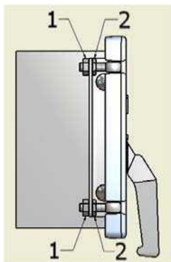
Rys. Instrukcja regulacji siły docisku drzwiczek
